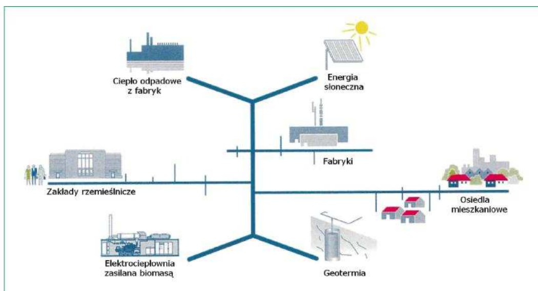
Rys. 7. Zasilenie gmin z ich zakładami rzemieślniczymi w ciepło oraz energię elektryczną na bazie różnorodnych odnawialnych nośników energii
