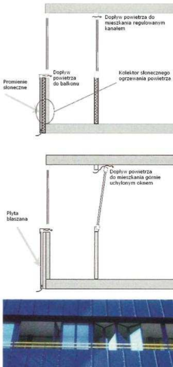
Rys. 2. Innowacje w ogrzewaniu wentylacyjnego powietrza poszczególnych mieszkań w starym bloku mieszkalnym poprzez oszklenie balkonów na południowej stronie i zainstalowaniu blachy absorbującej promieniowanie słoneczne wzdłuż balustrady
