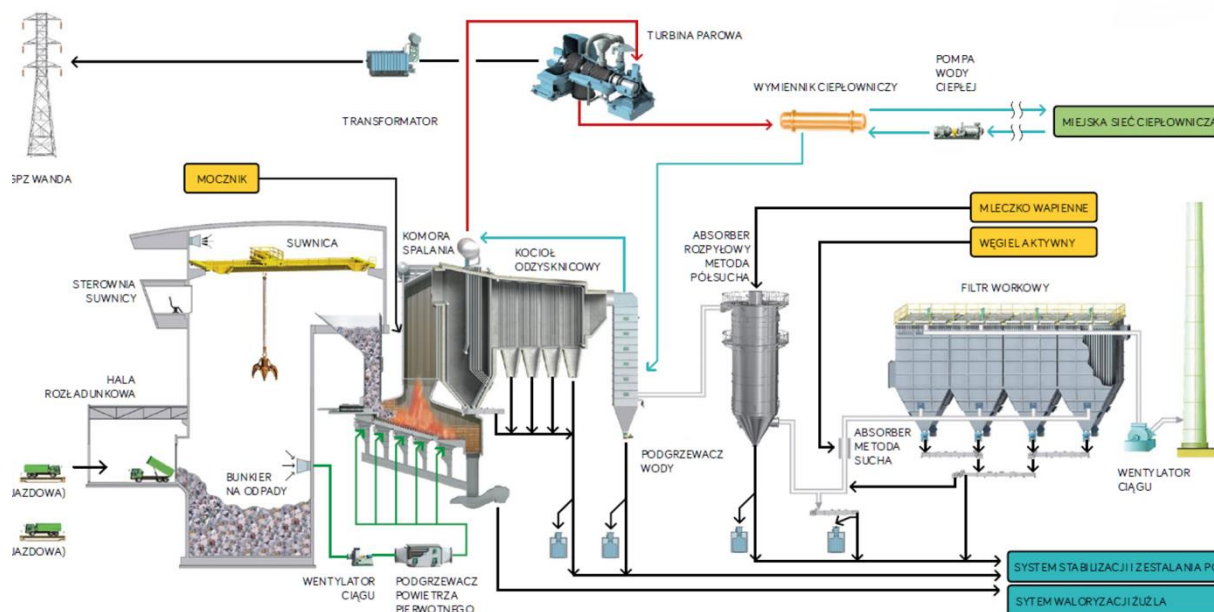
Rys. 7. Schemat technologiczno-funkcjonalny spalarni w Krakowie
